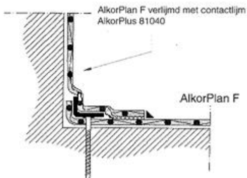
Lineaire kimfixatie mbv metaalfolieplaat+ verlijmd opstand
